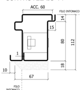
CONTROTELAIO TT
